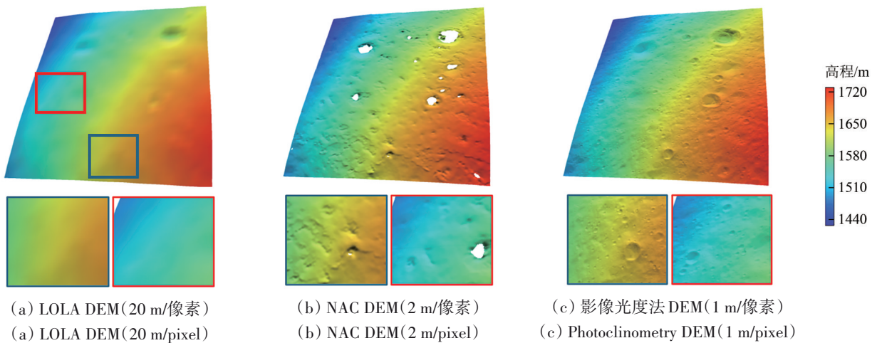
图8 实验区2 DEM对比以及矩形框中(LOLA DEM上)的局部细节
