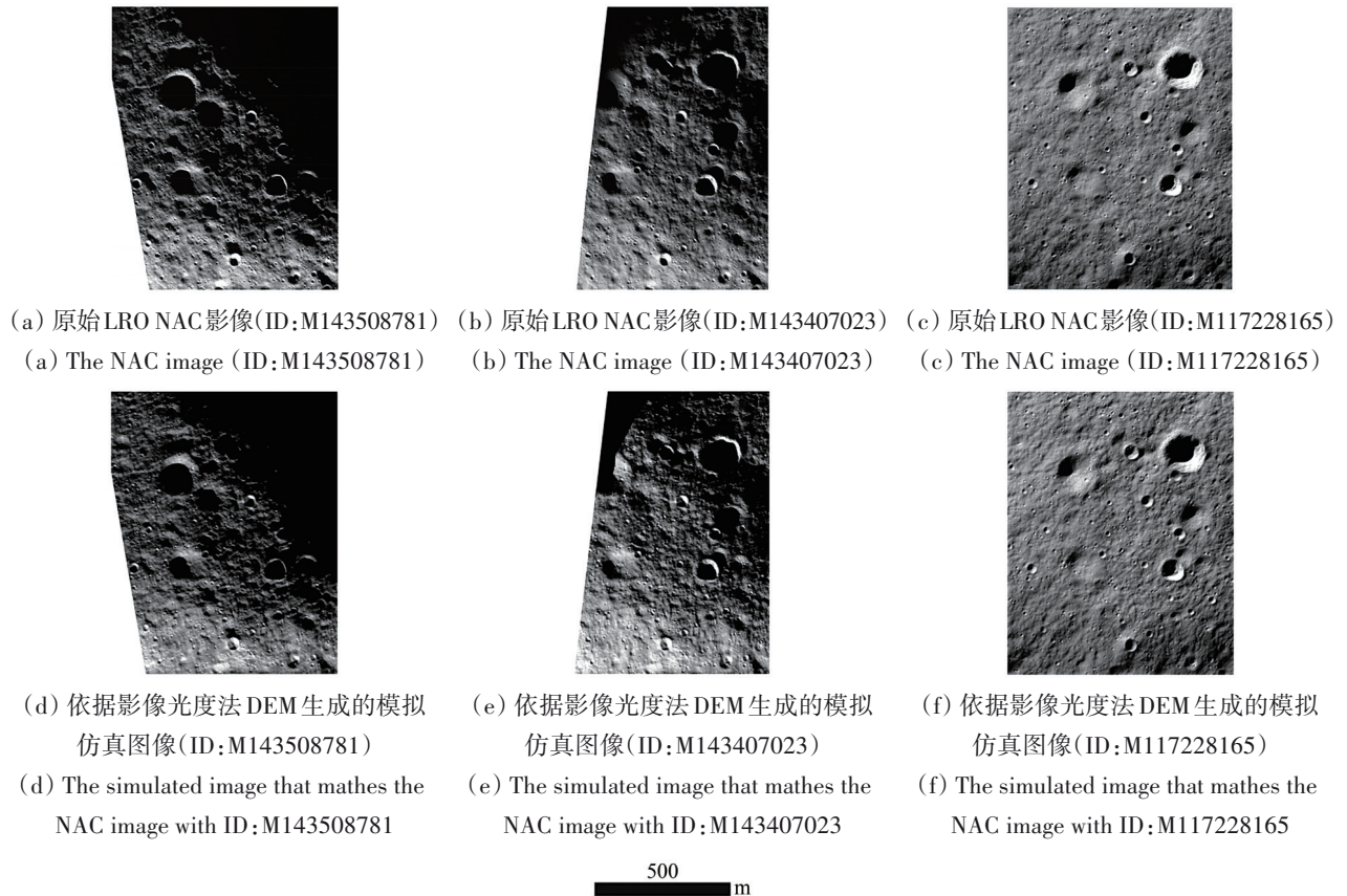
图 11 实验区 2 模拟仿真实验结果图 Fig. 11 Simulation results of test area 2
