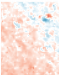
(d) LOLA DEM与LDEM差异图 (d) Difference map of LOLA DEM and LDEM
