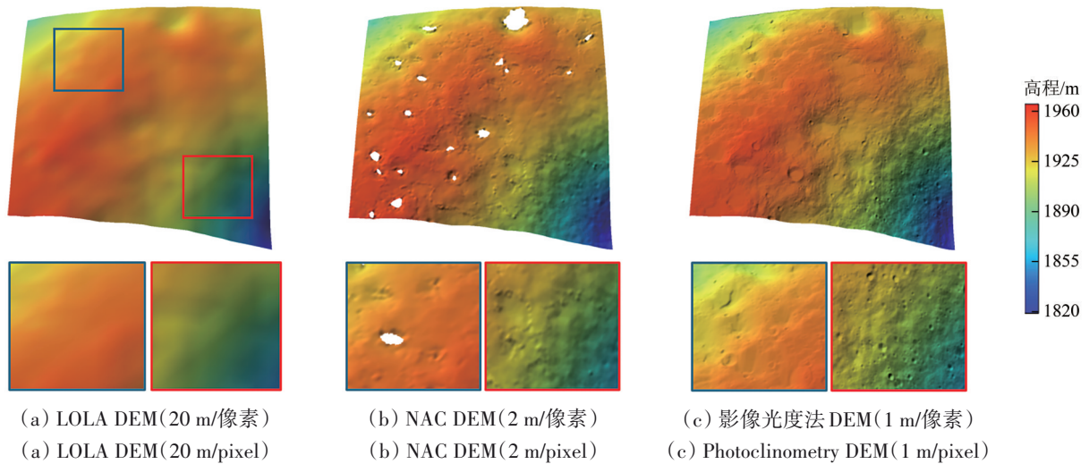
图4 实验区1 DEM对比以及矩形框中(图4 (a))的局部细节
