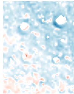
(b) LOLA DEM与摄影测量DEM差异图 (b) Difference map of LOLA DEM and photogrammetric DEM
