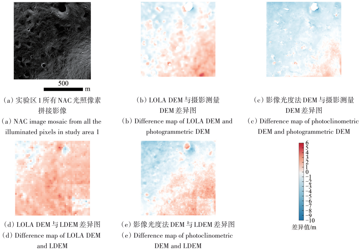
图5 实验区1 LOLA DEM、影像光度法DEM分别和摄影测量DEM、LDEM比较结果
