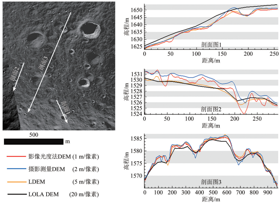
图 10 实验区 2 DEM 剖面图比较 Fig. 10 Profile comparison for study area 2
