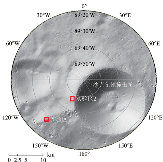
图2 实验区示意图
