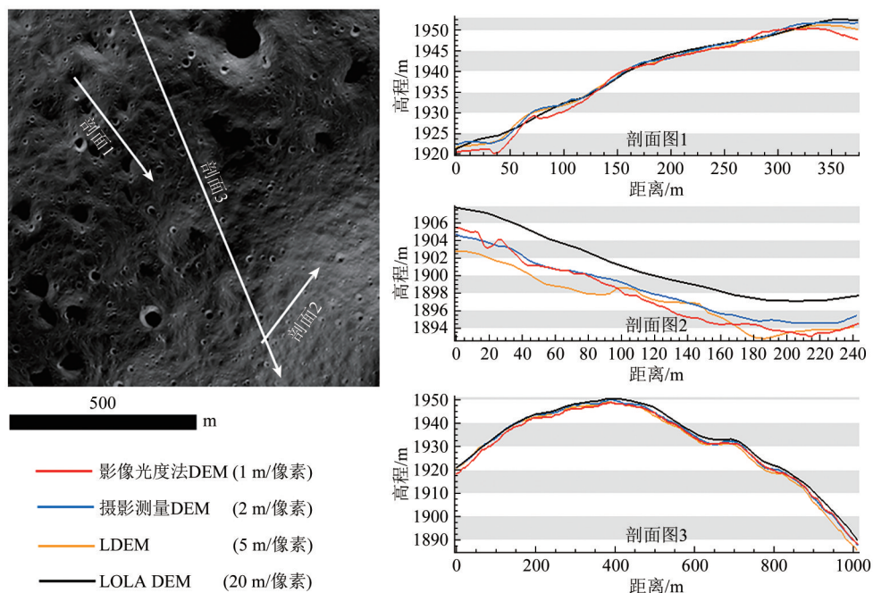
图6 实验区1 DEM剖面图比较
