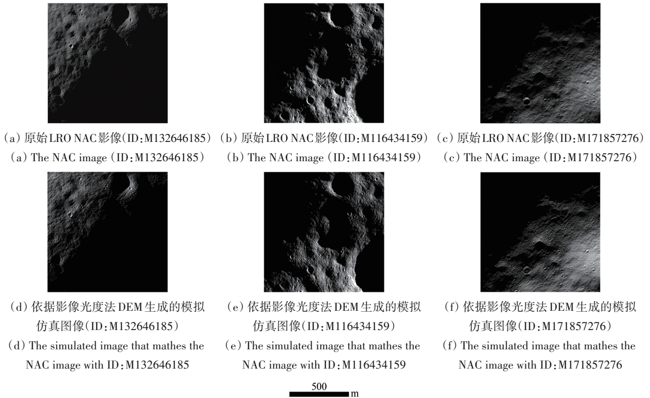
图7 实验区1模拟仿真实验结果图
