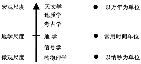
图 2 时间尺度谱和地学时间尺度 Fig 2 Temporal scale spectrum and geo-temporal scale
