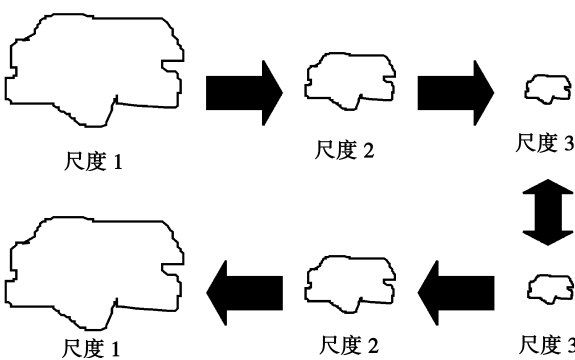
图 4 2 维欧氏空间尺度缩放示意图
