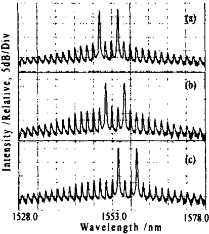
图 5 FP1 的双波长工作调节特性: (a) 工作波长峰值位于 1549.6nm 和 1554.6nm; (b) 工作波长峰值位于 1551.5nm 和 1556.4nm; (c) 工作波长峰值位于 1554.6nm 和 1559.6nm
