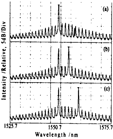
图 3 FP1 的输出光谱: (a) 单波长工作时 \lambda = 1549.6\text{nm} ; (b) 双波长工作时, 其中工作波长分别为 \lambda_1 = 1549.6\text{nm} 和 \lambda_2 = 1554.6\text{nm} ; (c) 双波长工作时, 其中工作波长分别为 \lambda_1 = 1549.6\text{nm} 和 \lambda_2 = 1559.6\text{nm}
