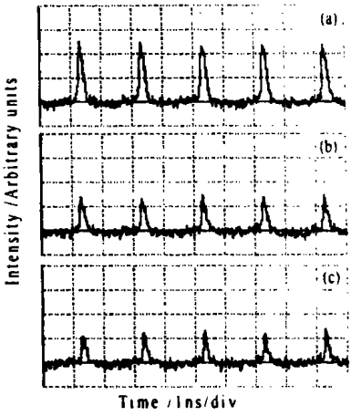
图 4 FP1 输出脉冲序列的时域特性: (a) 单波长工作时波长 \lambda = 1549.6\text{nm} 的脉冲序列; (b) 双波长工作时波长 \lambda_1 = 1549.6\text{nm} 的脉冲序列; (c) 双波长工作时波长 \lambda_2 = 1559.6\text{nm} 的脉冲序列
