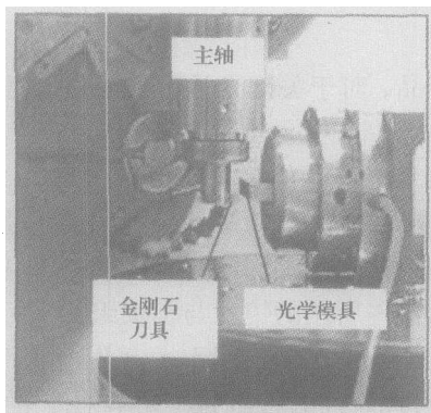
图4 “飞刀”铣削
