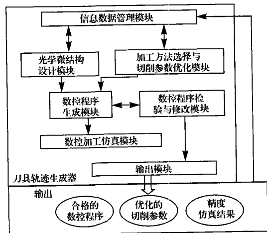
图 8 光学微结构刀具轨迹生成器的基本功能模块
