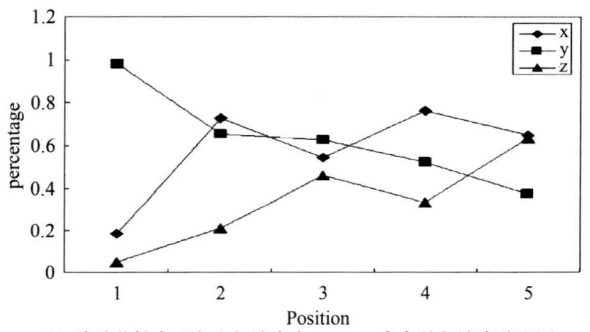
(c) 膝关节锁定下各点加速度在 x 、 y 、 z 方向的加速度分配图
