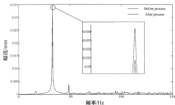
图 2 采集信号处理前后频谱图
