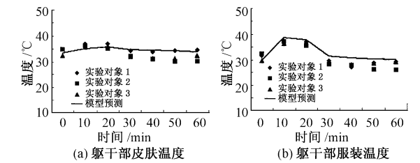
图2 着装部分(躯干)皮肤及服装温度理论预测与实验结果比较
