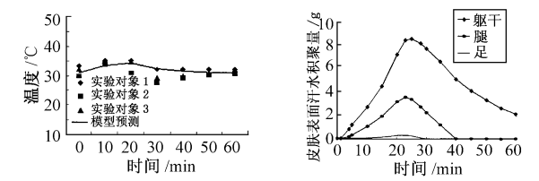
图3 裸露部分(臂)温度理论预测与实验结果比较
